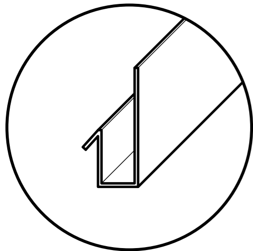
PERFIL INICIO INVISIBLE SIDING METAL
