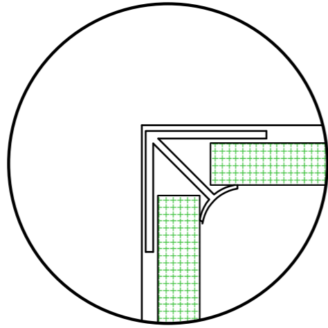
PERFIL ESQUINERO INTERIOR CIELO
