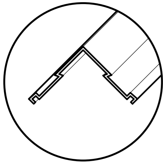
PERFIL ESQUINERO EXTERIOR SIDING METAL
