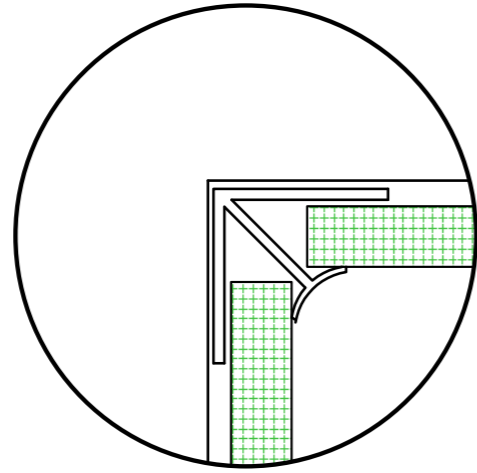
PERFIL ESQUINERO INTERIOR MURO
