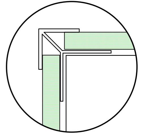
PERFIL ESQUINERO EXTERIOR CIELO
