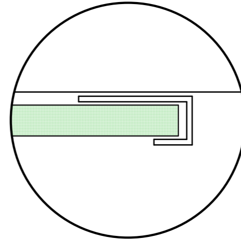
PERFIL J CIELO
